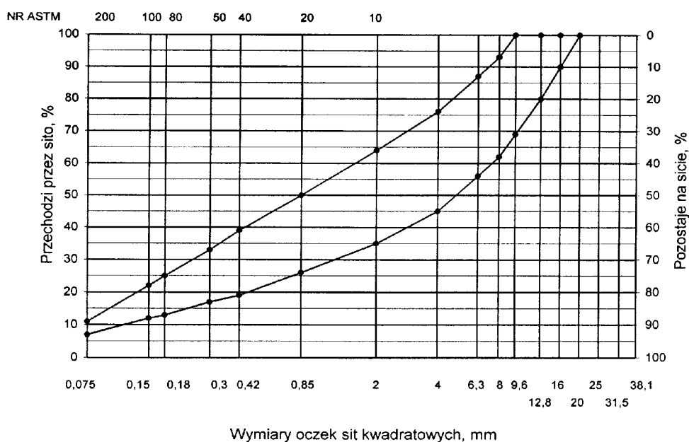
Rys. 1. Krzywe graniczne uziarnienia mieszanki mineralnej AC od 0 do 16mm, od 0 do 12,8 mm do warstwy ścieralnej nawierzchni drogi o obciążeniu ruchem KR1 lub KR2
